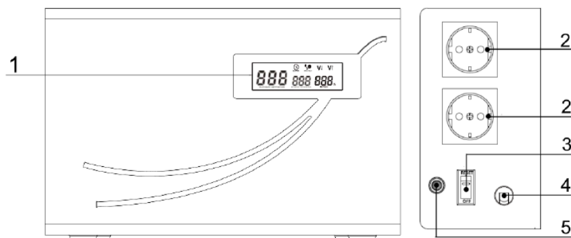
Рисунок 2. Внешний вид стабилизаторов напряжения SMARTWATT AVR SLIM 1500-2000VA. Описание элементов приводится в таблице 2.
